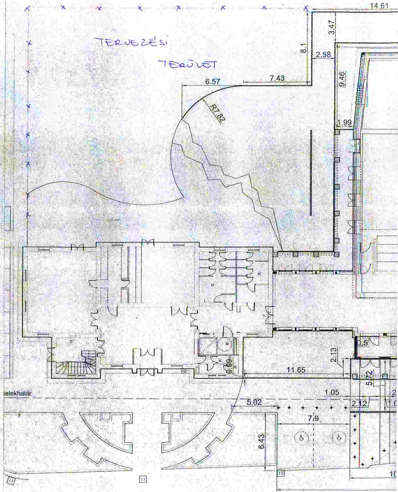
Burkolati minőségek átnézeti terve M=1:250
