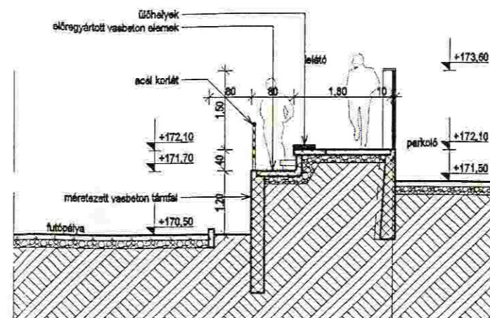
EGYSOROS LELÁTÓ METSZETE
