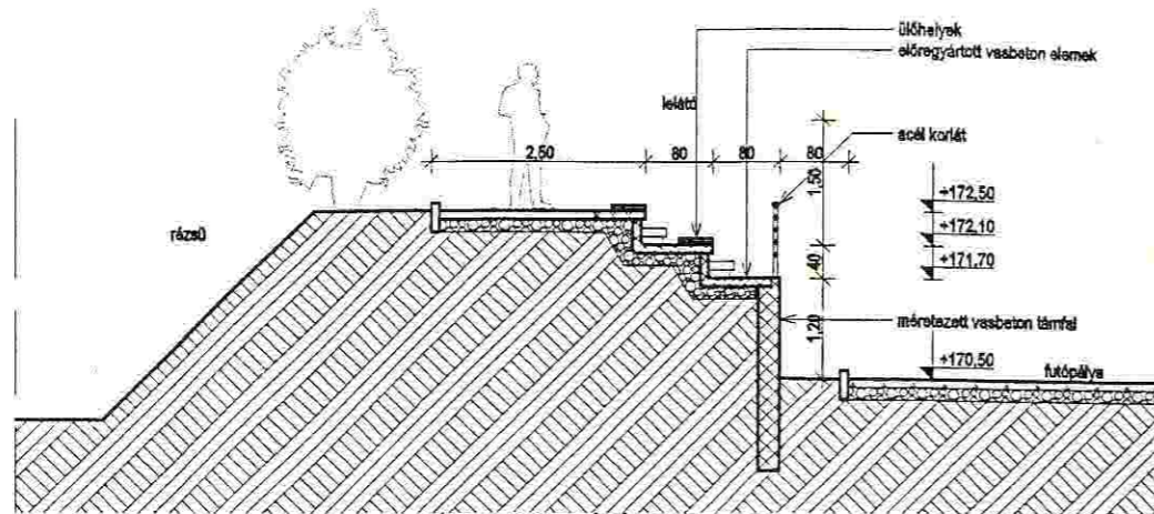
KÉTSOROS LELÁTÓ METSZETE
