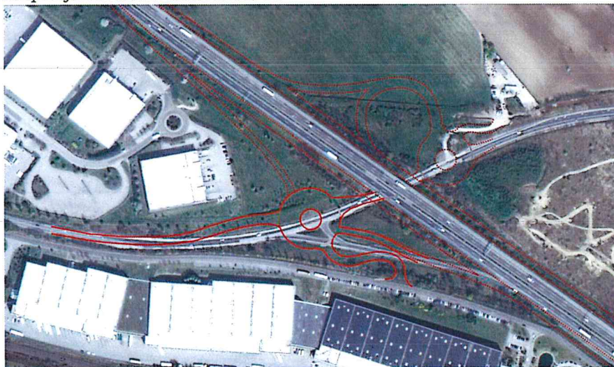
20. ábra: Támogatott megoldás a Verebely utcai átkötés, ill. az M1 - 1. sz. főút csomópontjának távlati átalakításánál
