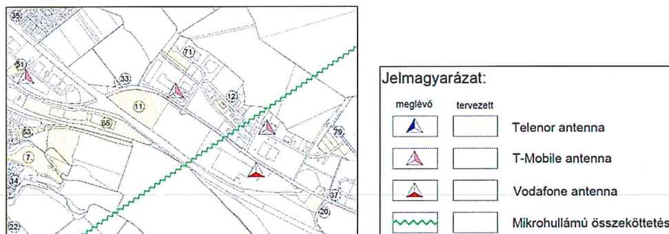
30. ábra: A tervezési terület környezetében található hírközlési berendezések és mikrohullámú összeköttetés vonala
