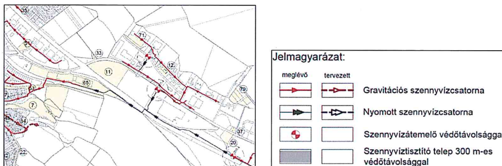
25. ábra: A CTP Management Hungary Kft. által megvásárolni szándékozott 7724/66-os hrsz.-ú ingatlan érintő szennyvízelvezető rendszer
