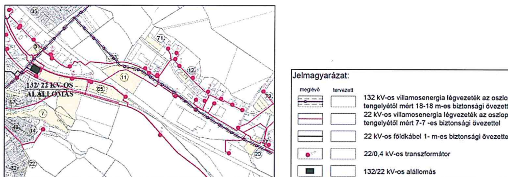
28. ábra: A tárgyi telephelyet érintő elektromos hálózat
