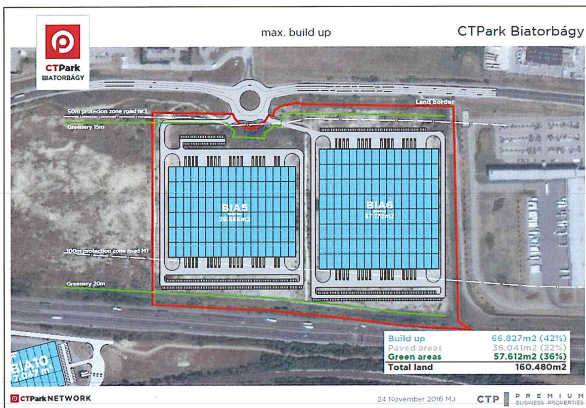
17. ábra: A Biatorbágy, 7724/66-os hrsz.-ú ingatlan helyszínrajza a tervezett csarnokok ábrázolásával 42%-os beépítettség esetén
