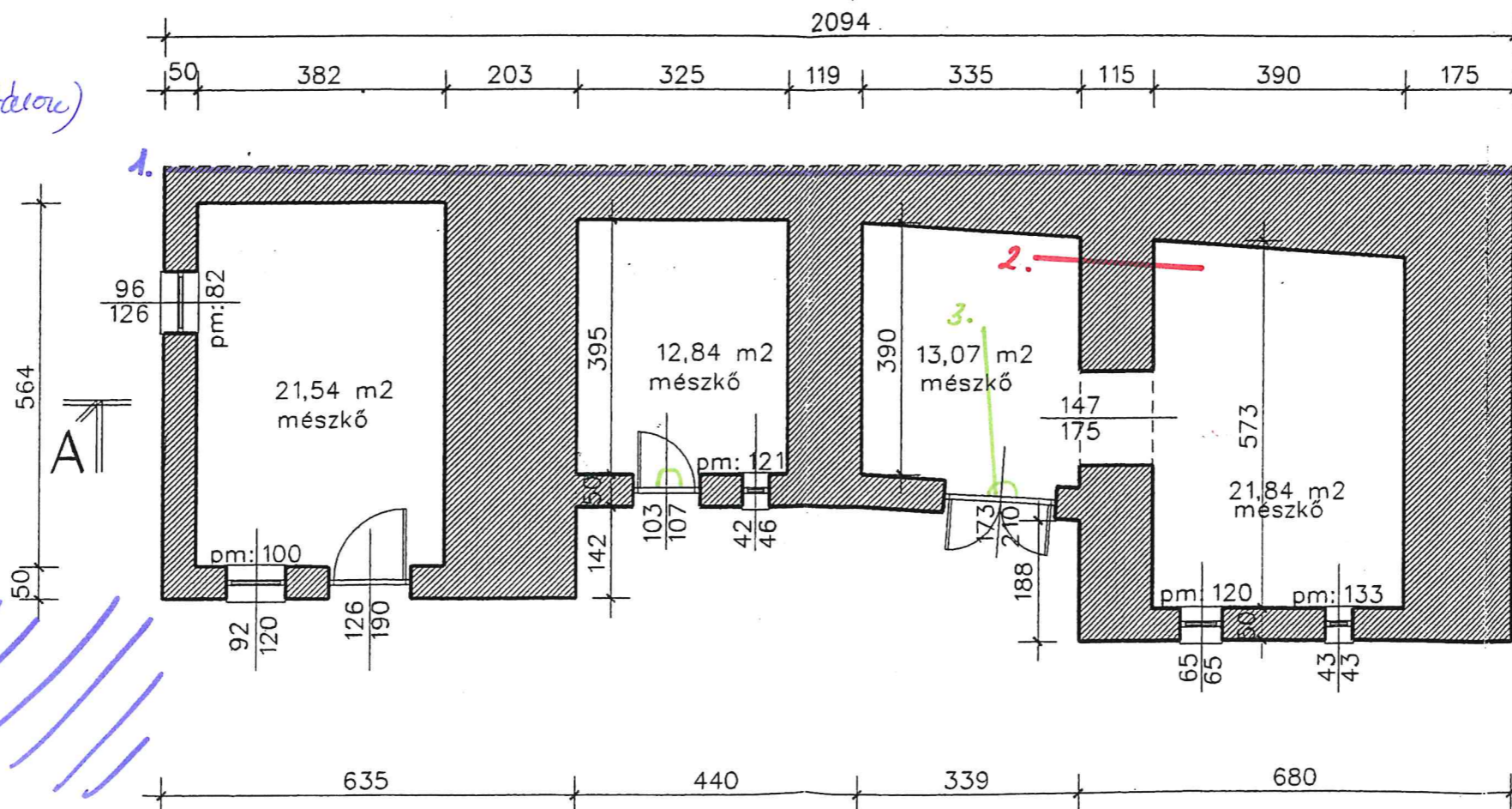
ALAPRAJZ, METSZET M 1:100
