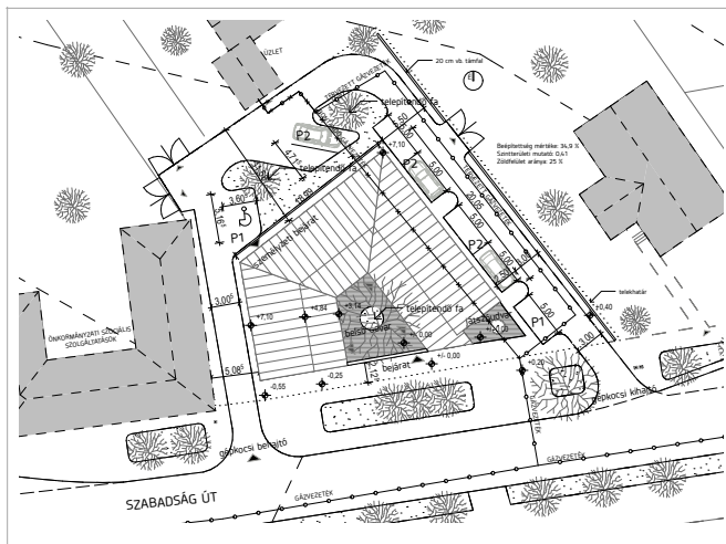
Korábbi terv helyszínrajza
