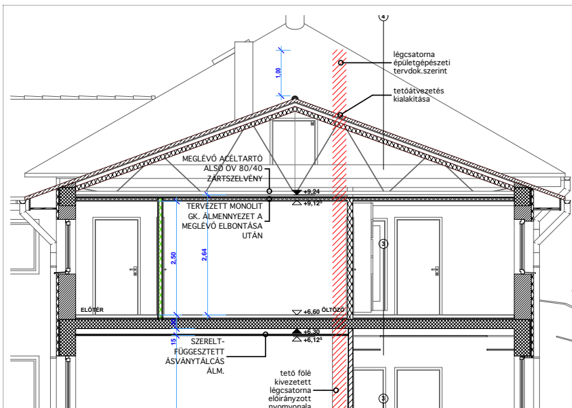
A 2. emelet jellemző metszete
