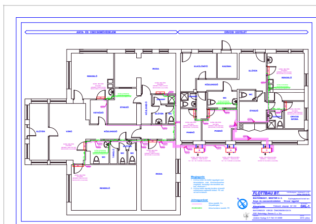
Gépészeti felújítás terve, balra az eredeti épületrész
