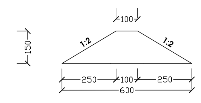
TERVEZETT RÉZSÚ A - A MINTAMETSZETE - M = 1:100
