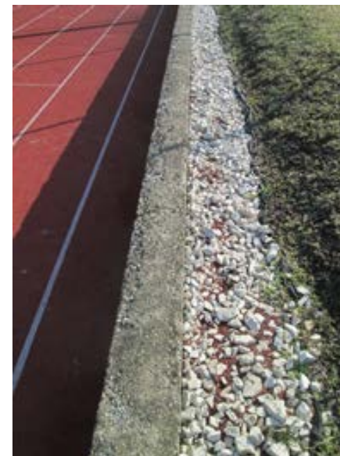
Csapadékvíz elvezetés és burkolatok a sporttelepen
